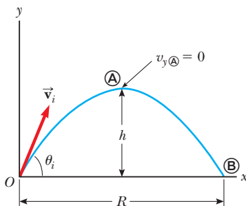
Figura 4.9 Proyectil lanzado sobre una superficie plana desde el origen en t_i = 0 con una velocidad inicial \vec{v}_i . La altura máxima del proyectil es h y el alcance horizontal es R . En A, el máximo de la trayectoria, la partícula tiene coordenadas (R/2, h) .
